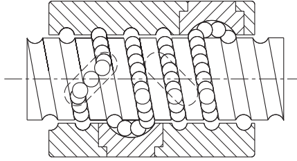
圖 1.6.1 U, I 型螺帽圖
