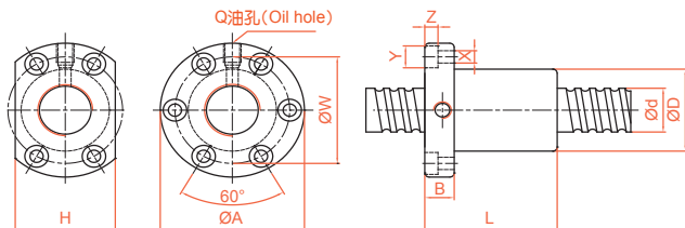
GI 轉造級系列規格尺寸表
