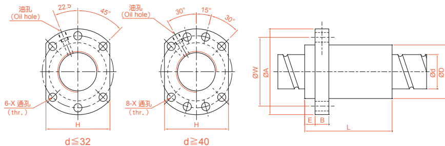
GH (DIN 69051 FORM B) 精密研磨級系列規格尺寸表
