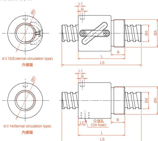
CH 轉造級系列規格尺寸表
