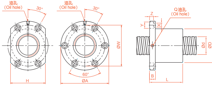
GV 精密研磨級系列規格尺寸表
