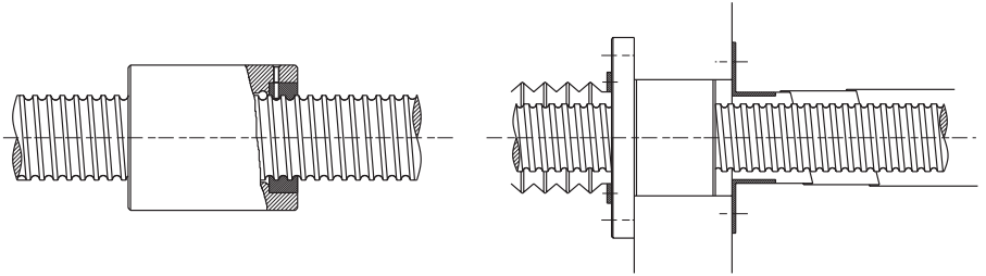
圖 1.10.2 防塵機構
