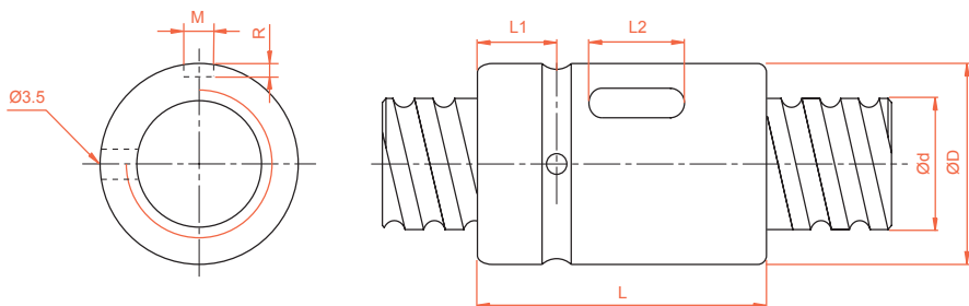
CS 轉造級系列規格尺寸表
