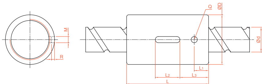
CN 精密研磨級系列規格尺寸表
