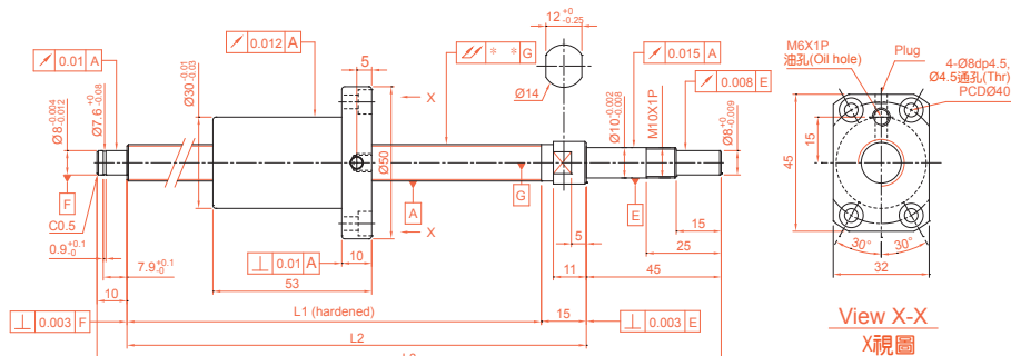
XGVR01210-01 精密研磨級系列規格尺寸表 ( 研磨級軸端完成品 )
