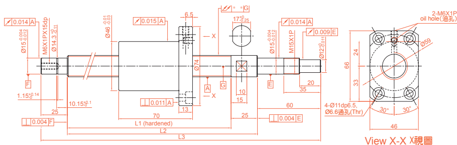
XGVR02020-00 精密研磨級系列規格尺寸表 (研磨級軸端完成品)
