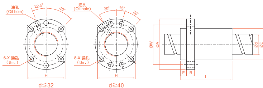
GH (DIN 69051 FORM B) 轉造級系列規格尺寸表
