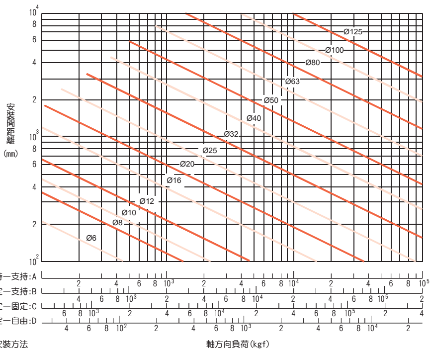
圖 1.4.16 挫屈之容許壓縮負荷
