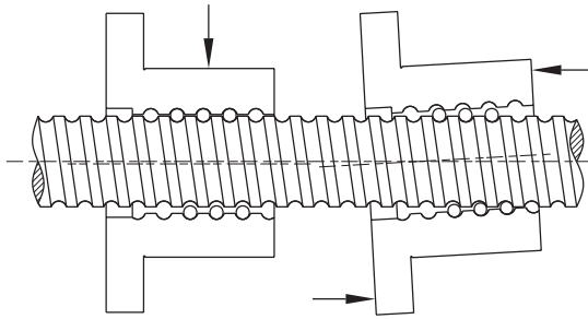
圖 1.10.3 偏荷重
