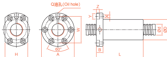
GSI/GDI 精密研磨級系列規格尺寸表
