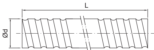
圖 2.3.1 螺桿示意圖
