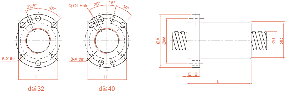
GA 精密研磨級系列規格尺寸表
