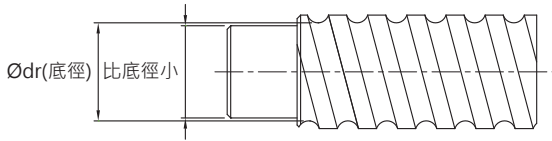
圖 1.10.4 出牙—內循環軸端必要條件
