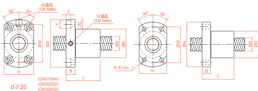
GK 精密研磨級系列規格尺寸表
