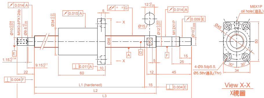
XGVR01520-01 精密研磨級系列規格尺寸表 (研磨級軸端完成品)
