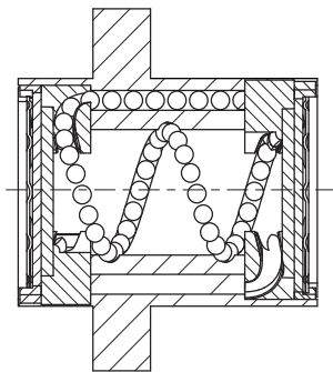
圖 1.6.4 Y, H, A 型螺帽圖
