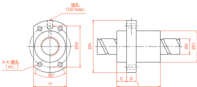
GY 轉造級系列規格尺寸表
