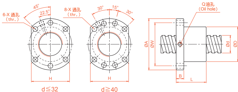
GU (DIN 69051 FORM B) 轉造級系列規格尺寸表
