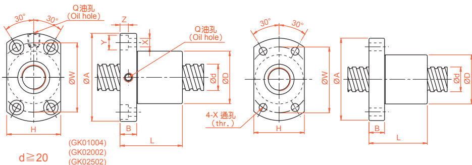
GK 轉造級系列規格尺寸表
