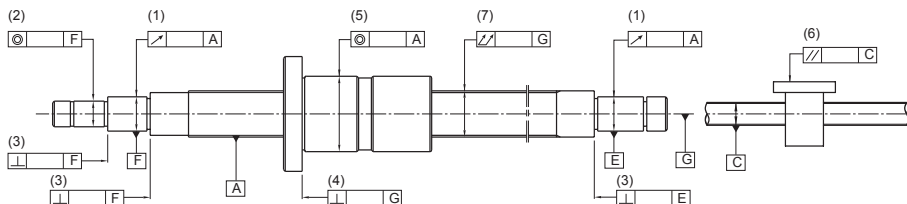
圖 1.3.2 滾珠螺桿安裝部位的精度
