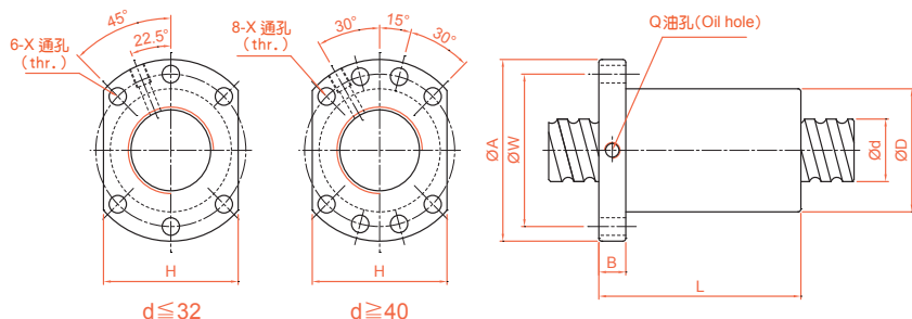
GSU/GDU (DIN 69051 FORM B) 精密研磨級系列規格尺寸表
