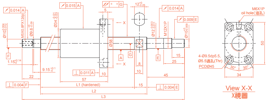
XGVR01510-00 精密研磨級系列規格尺寸表 (研磨級軸端完成品)
